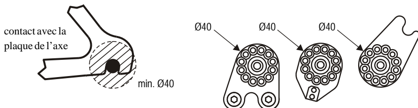
Image 1: Surface interne d'appui plate sur la patte gauche et les trois formes de plaques de l'axe.
