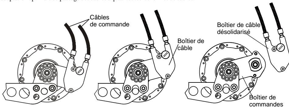
Possibilités de montage en version EX avec plaque de l'axe standard et bras de couple.
